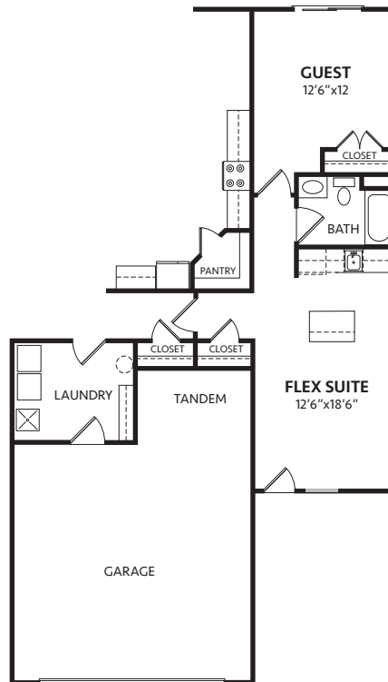
OPTIONAL FLEX SUITE
